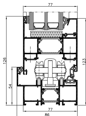
Przekrój dolny drzwi z uszczelnieniem przymykowym
